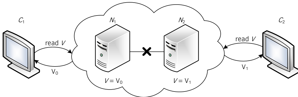
C.2. ábra. A V adegység nem konzisztens, a C_1 és a C_2 kliensek eltérő értéket látnak
