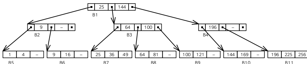
3.7. ábra. Egy adatstruktúra B*-fa szervezés esetén
