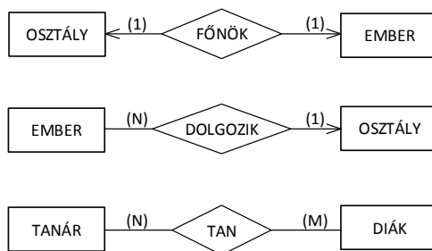
4.2. ábra. Kapcsolatok funkcionalitásának egy ábrázolása az ER-diagramoknál
