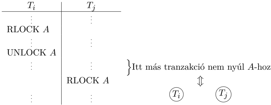
10.4. ábra. Precedenciagráf READ \dots READ szekvencia esetén az R/W tranzakciómodellben – természetesen az ütemezés másik szekvenciája miatt keletkezhet él T_i és T_j között
