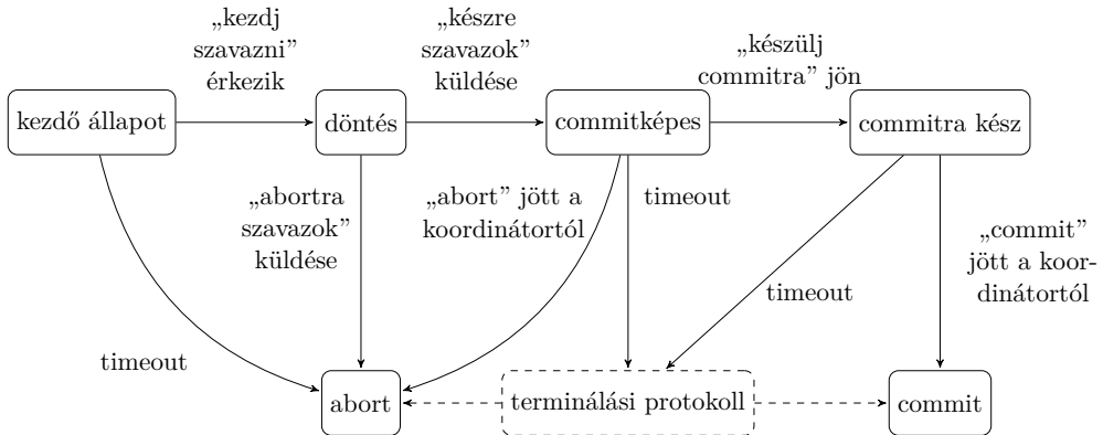
11.5. ábra. Egy résztvevő fontosabb állapotai a 3PC protokollban
