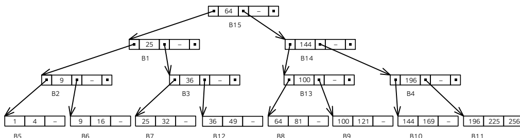
3.8. ábra. A B*-fa a 32 kulcsú rekord beszúrása után
