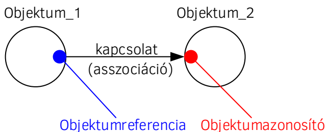
8.2. ábra. Az objektumazonosító és az objektumreferencia
