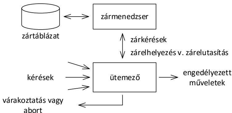
10.1. ábra. A konkurens működés elemei zár alapú tranzakciókezelés esetén
