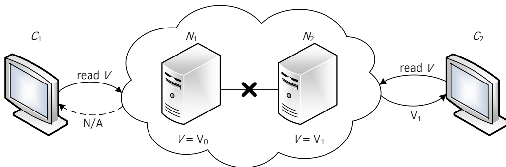
C.3. ábra. A C_1 kliens számára a V adegység nem elérhető
