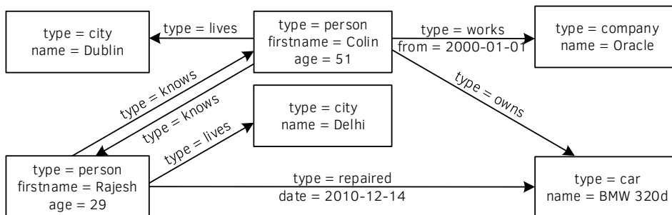
C.13. ábra. Tulajdonsággráf
