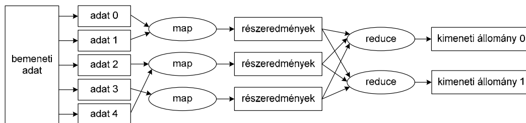
14. ábra: A MapReduce fázisai
