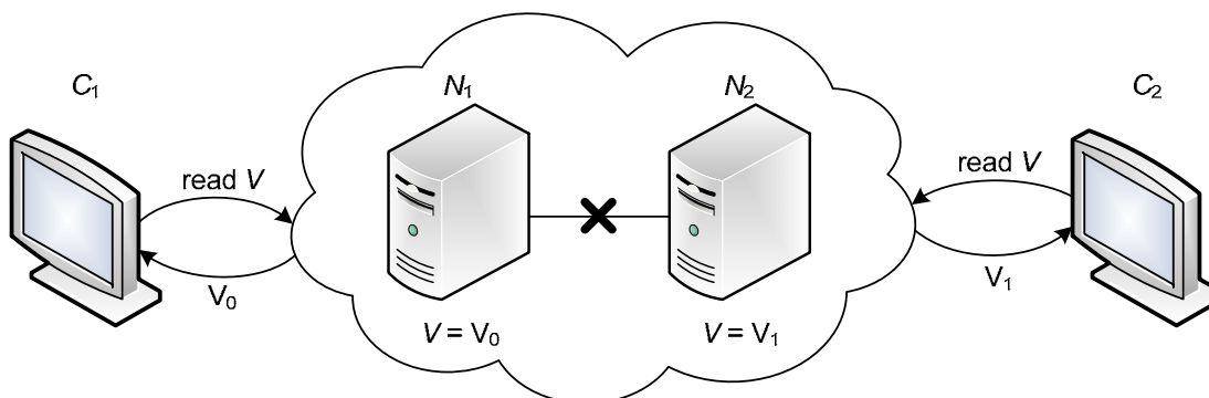
2. ábra: A V adategység nem konzisztens, a C_1 és a C_2 kliensek eltérő értéket látnak
