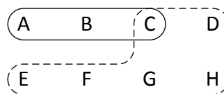
7. ábra: Írási (szaggatott vonal) és olvasási testületek ( N = 8 , R = 3 , W = 6 )
