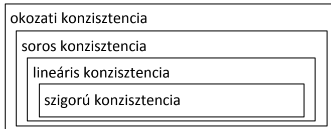
6. ábra: Adatközpontú konzisztenciamodellek. A szűkebb halmazok modelljei erősebb garanciákat nyújtanak.
