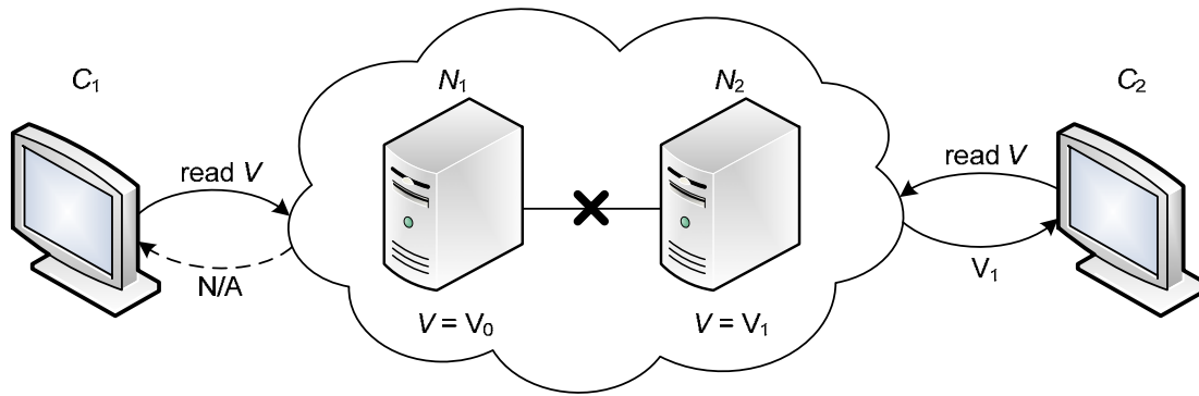
3. ábra: A C_1 kliens számára a V adataegység nem elérhető
